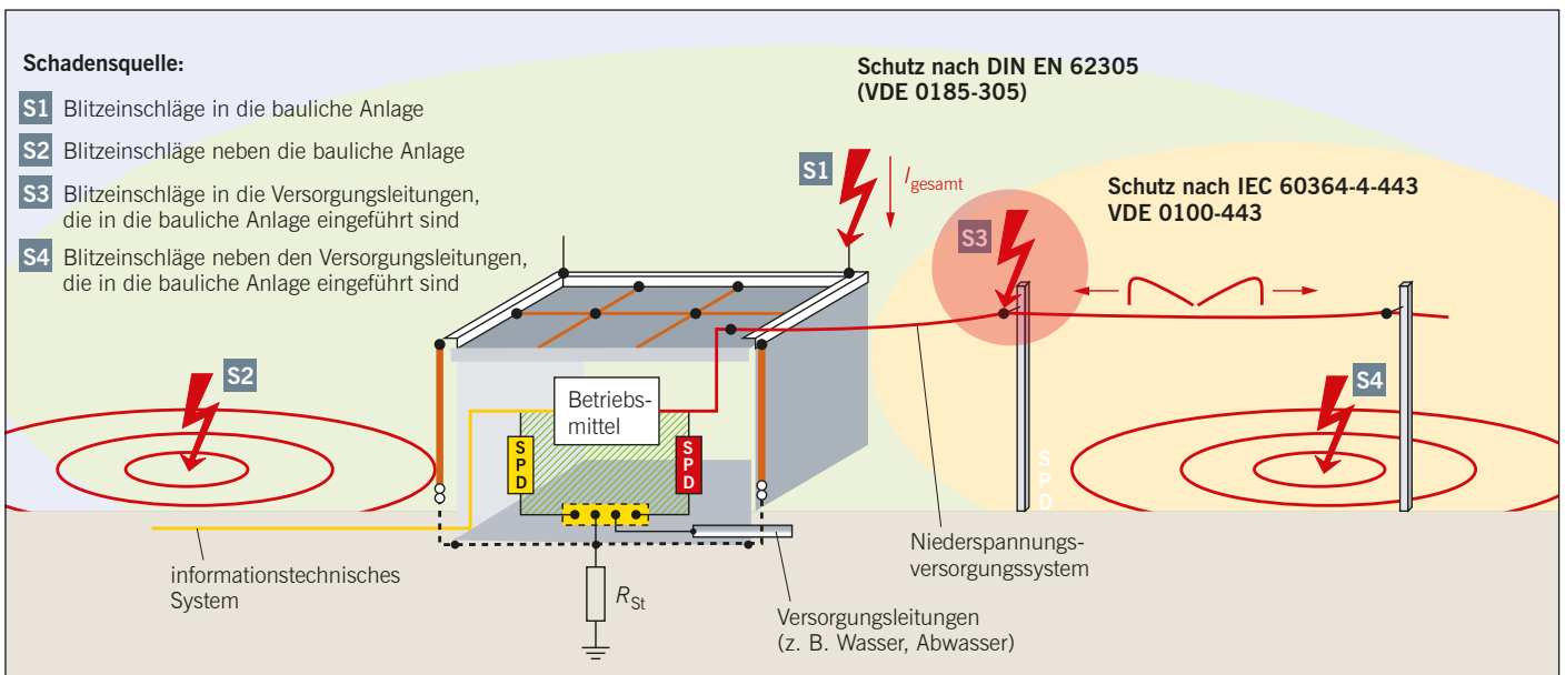
2 Zuordnung der Schadensquellen S1 bis S4 - Direkte Blitzeinschläge in Versorgungsleitungen im Anwendungsbereich DIN VDE 0100-443
