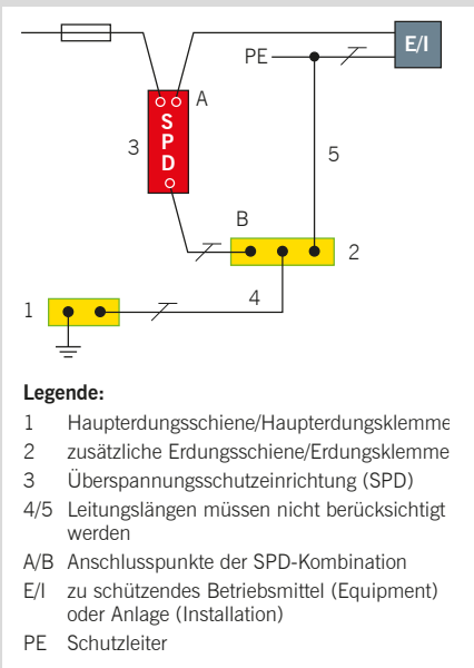
16 Optimierung der Anschlusslänge eines SPDs
