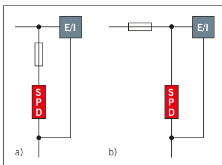
13 Anordnungsmöglichkeiten des Überstromschutzes bei SPDs
