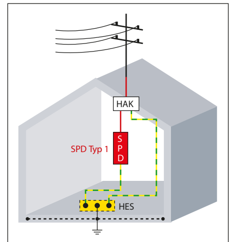
1 Überspannungsschutz bei Gebäuden ohne äußeres Blitzschutzsystem, aber mit Einspeisung über eine Niederspannungsfreileitung
